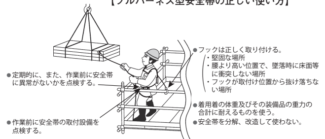
【フルハーネス型安全帯の正しい使い方】
