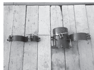
開発した取付装置の写真
