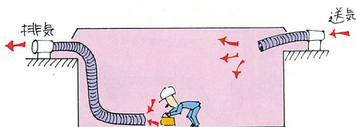
●地下室の換気
