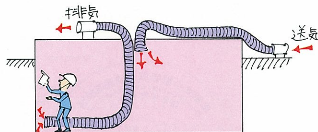
●マンホールからの換気
