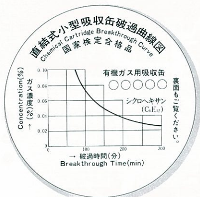
隔離式吸収缶破過時間表の例
