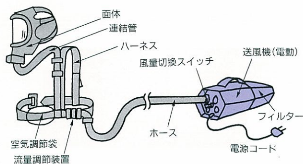
電動送風機形送気マスク
