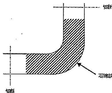
図 配管ニル部の事例
